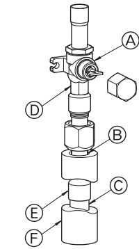
(A) Kapama vanası (B) Conta bölümü (C) İç boru (D) Çift gerçi kısmı (E) Bağlantı borusu (F) Boru kapağı
