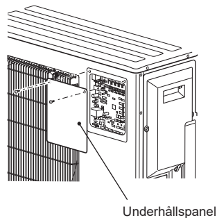
Underhållspanel
