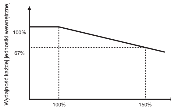
Stosunek łącznej wydajności jednostek wewnętrznych do wydajności jednostki zewnętrznej
