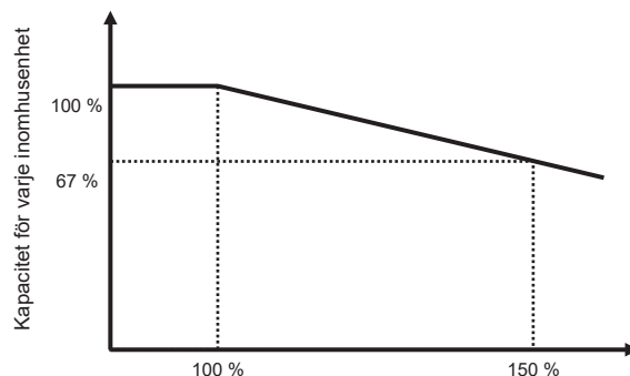
Förhållande mellan inomhusenheternas totala kapacitet och utomhusenhetens kapacitet Drift när den totala kapaciteten för inomhusenheterna i drift överstiger utomhusenhetens kapacitet.
