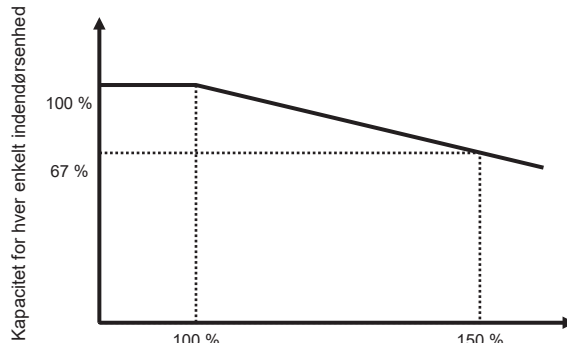
Forholdet mellem indendørsenhedernes samlede kapacitet udendørsenhedens kapacitet Drift, når de aktive indendørsenheders samlede kapacitet er større end udendørsenhedens kapacitet.
