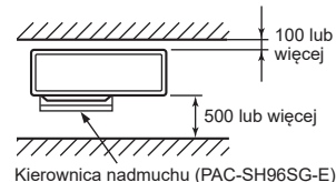
Kierownica nadmuchu (PAC-SH96SG-E)
