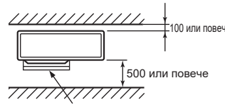
Направляващо устройство на изхода за въздух (PAC-SH96SG-E)
