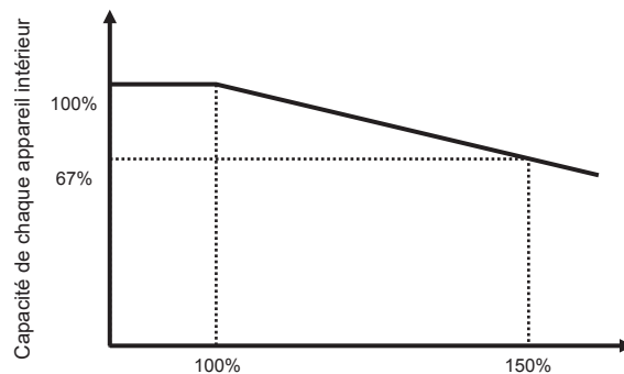
Rapport entre la capacité totale des appareils intérieurs et la capacité de l'appareil extérieur Fonctionnement lorsque la capacité totale des appareils intérieurs en fonctionnement est supérieure à celle de l'appareil extérieur.
