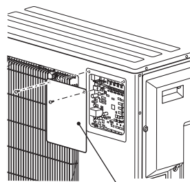
Vedlikeholdspaneel
