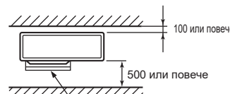
Направляващо устройство на изхода за въздух (MAC-856SG)
