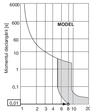
Valoarea nominală a intensității curentului de declanșare (x) Model de grafic
