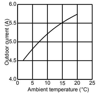
MUZ-SF42VE MUZ-SF42VEH
